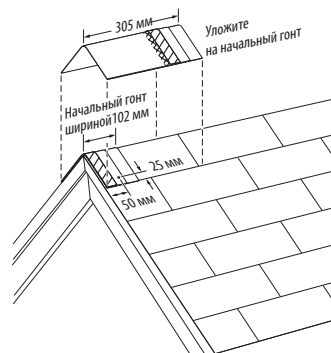
Рис. 15-20. Уложите целый покрывающий гонт на начальный гонт.
