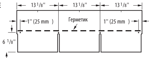
Рис. 10-3. Прибивайте каждый целый гонт четырьмя гвоздями.
