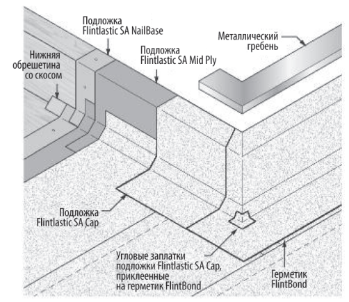
Рис. 5-43. Наружный угол в трёхслойной системе.
