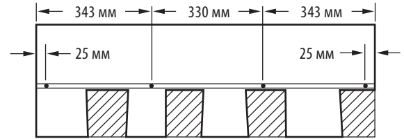
Рис. 12-4. Прибивайте каждый целый гонт четырьмя гвоздями.
