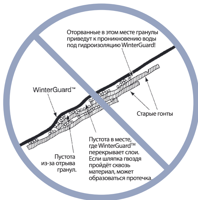
Рис. 5-4. Проблемы, возникающие при укладке WinterGuard на крышу.
