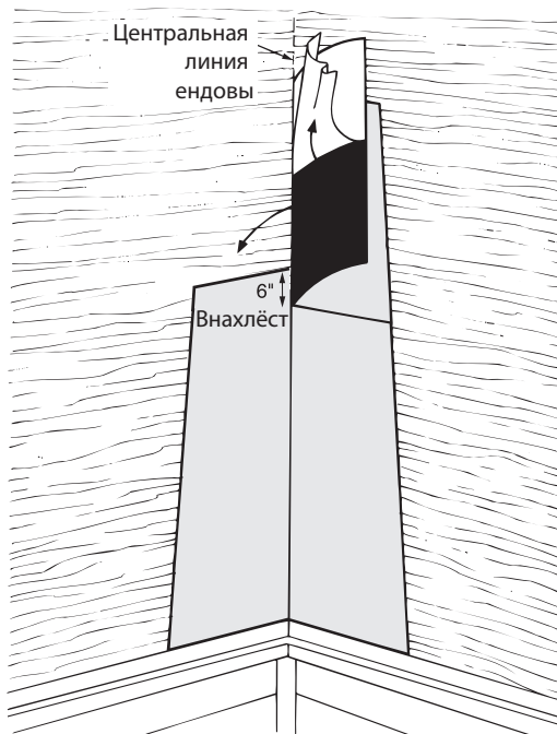
Рис. 5-9. Укладка в ендовах методом «задиранья и прижима» с участием двух рабочих.
