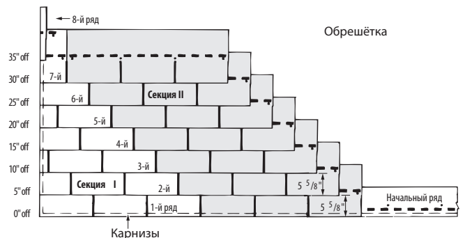
Рис. 10-15. Восьмирядный метод укладки с отрезанием по 12,7 см и монтажом с уступом по диагонали.
