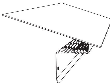
Рис. 7-15А. При монтаже на дома без софитов вентилируемый капельник сочетается в себе с входными жалюзийными отверстиями.
