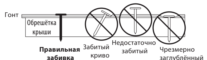
Рис. 14-2. Правильная и неправильная забивка гвоздей.
