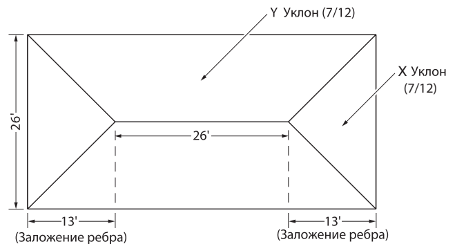
Рис. 3-5. Вид обычной вальмовой крыши в плане.
